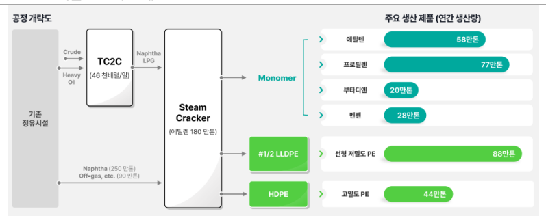
도표 6. 샤힌 프로젝트 개요
