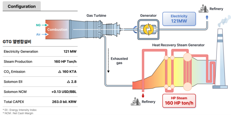
도표 8. GTG (Gas Turbine Generator) 프로젝트 개요
