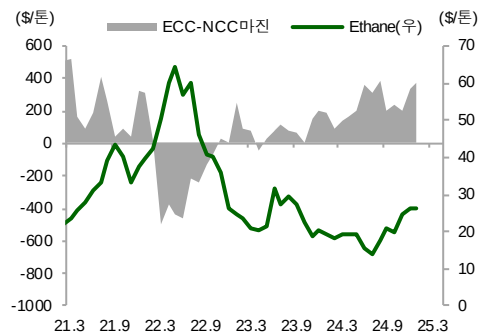
도표 106. 에탄 가격과 ECC-NCC 마진 추이
