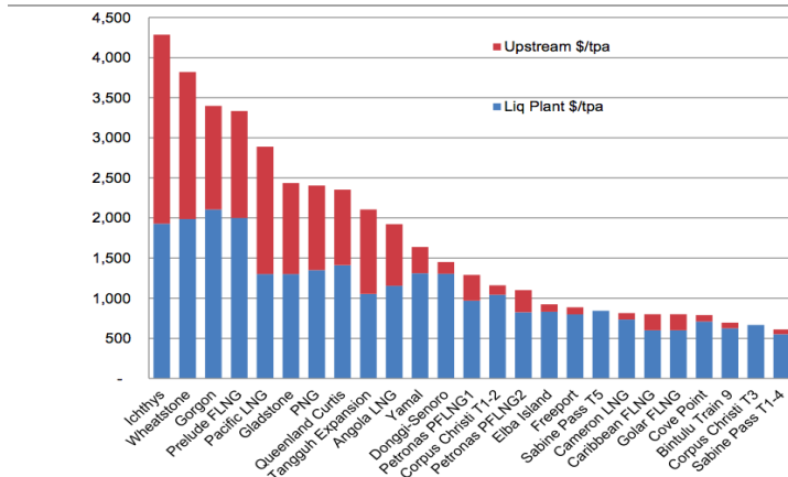
도표 13. LNG 프로젝트 개발 비용
